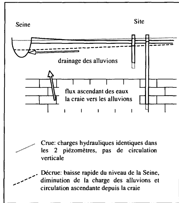
Figure 4. Comportement des différentes nappes lors d'une décrue de la Seine.
